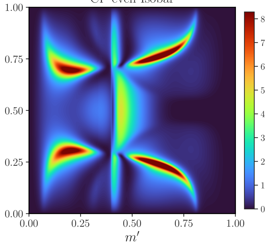
CP-even Isobar
