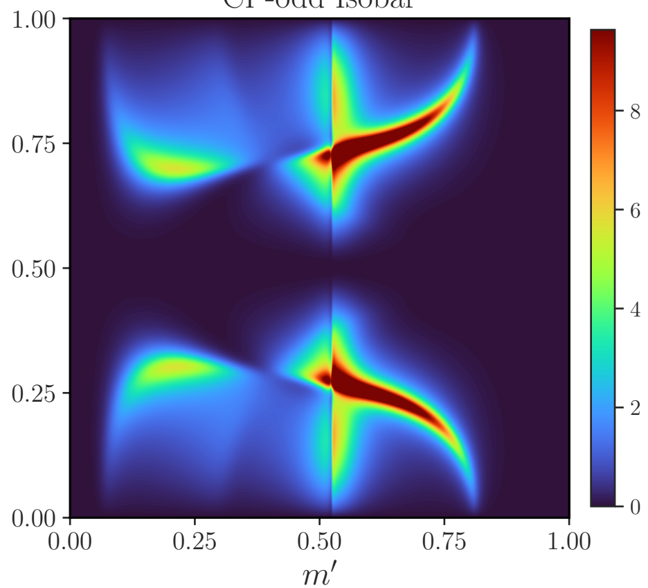
CP-odd Isobar
